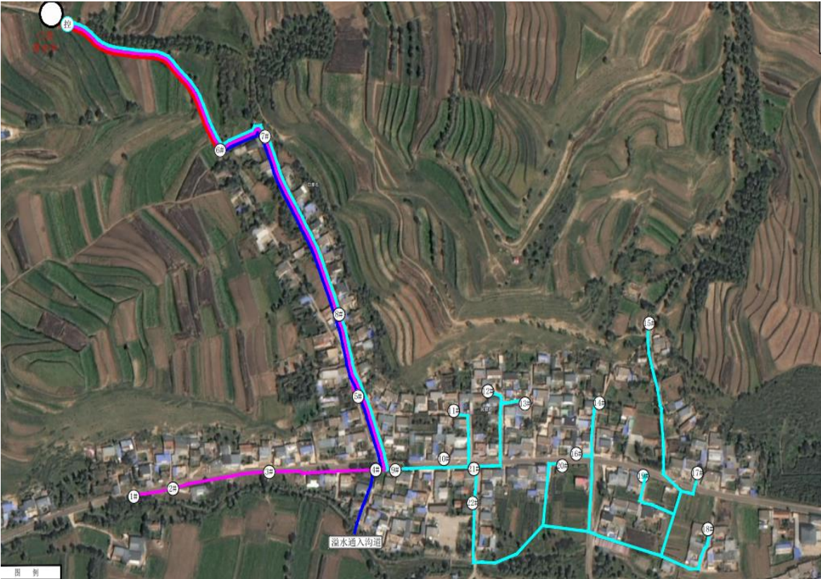
民联村管网布置图
