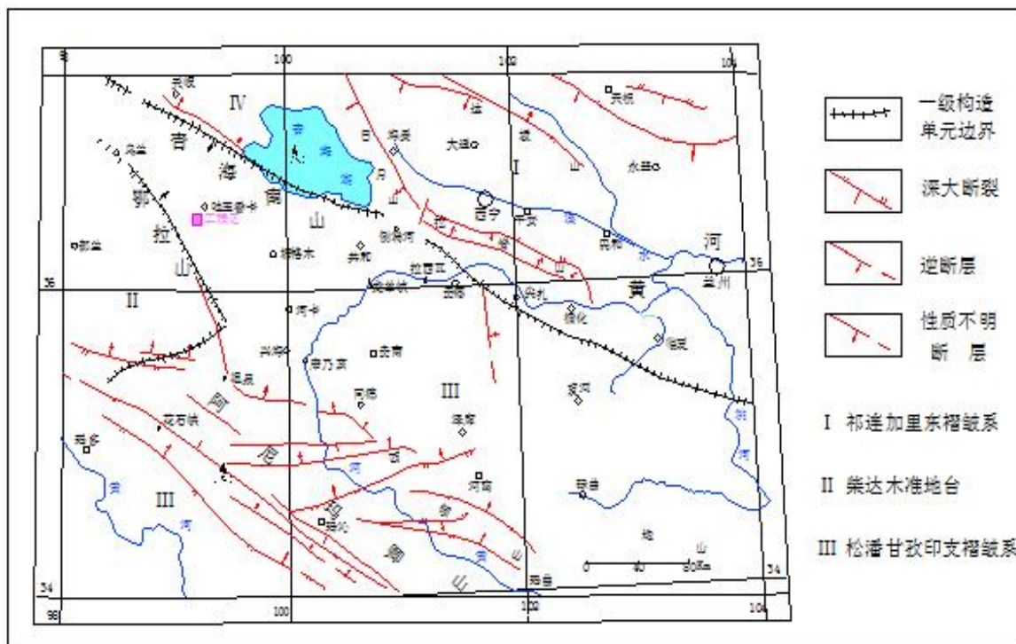
图 2-1 区域大地构造略图
